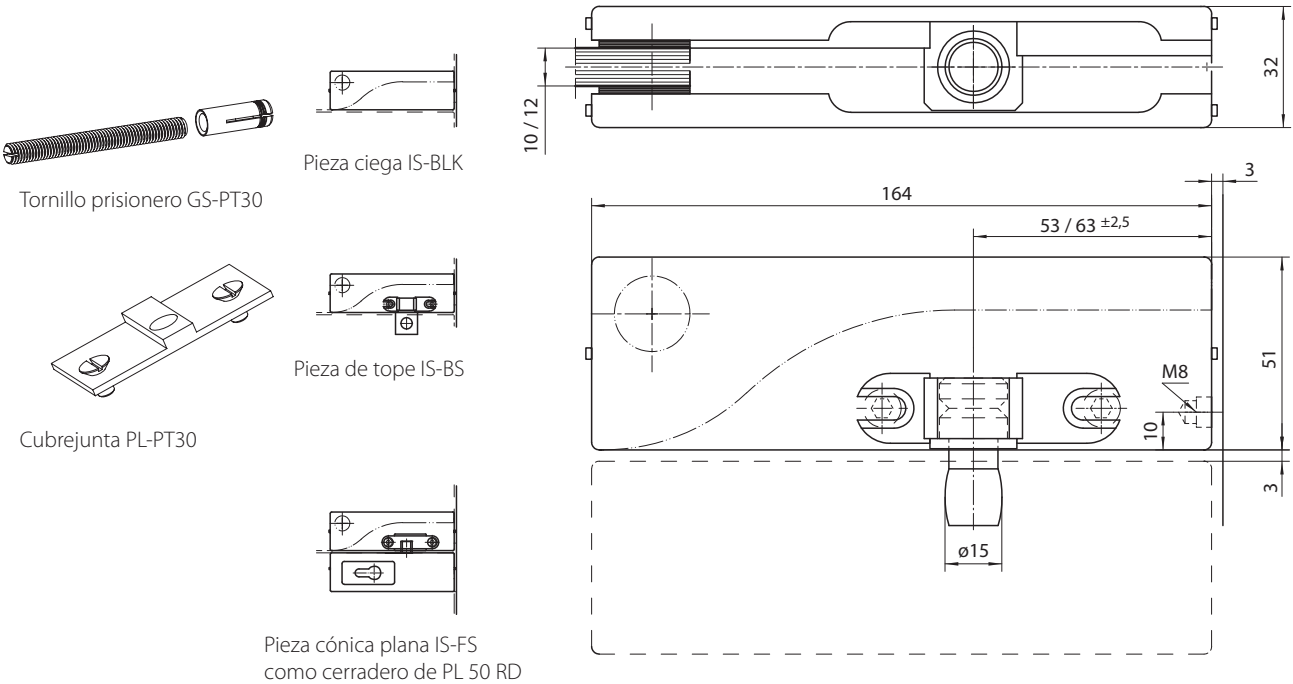
Dibujo nº 91905-1-0104
