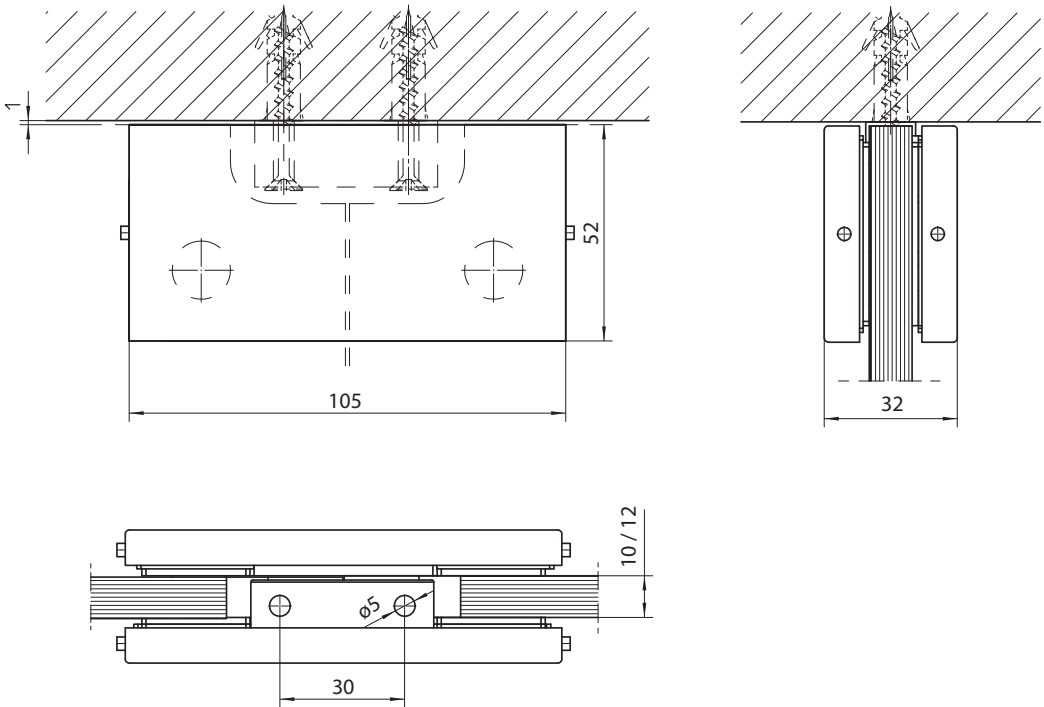
Dibujo nº 91905-1-0115
