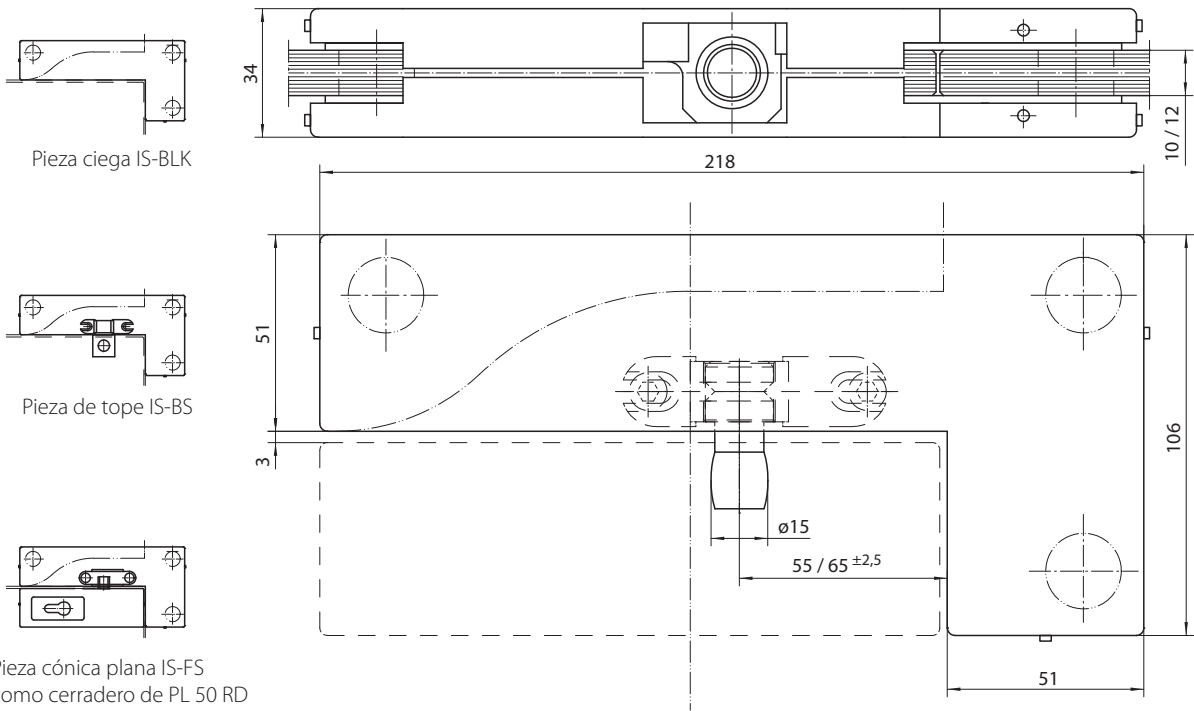
Dibujo nº 91905-1-0106
