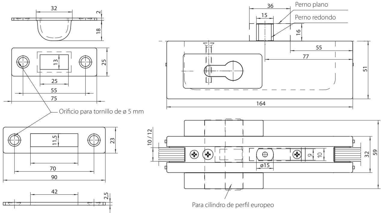
Dibujo nº 91905-1-0122
