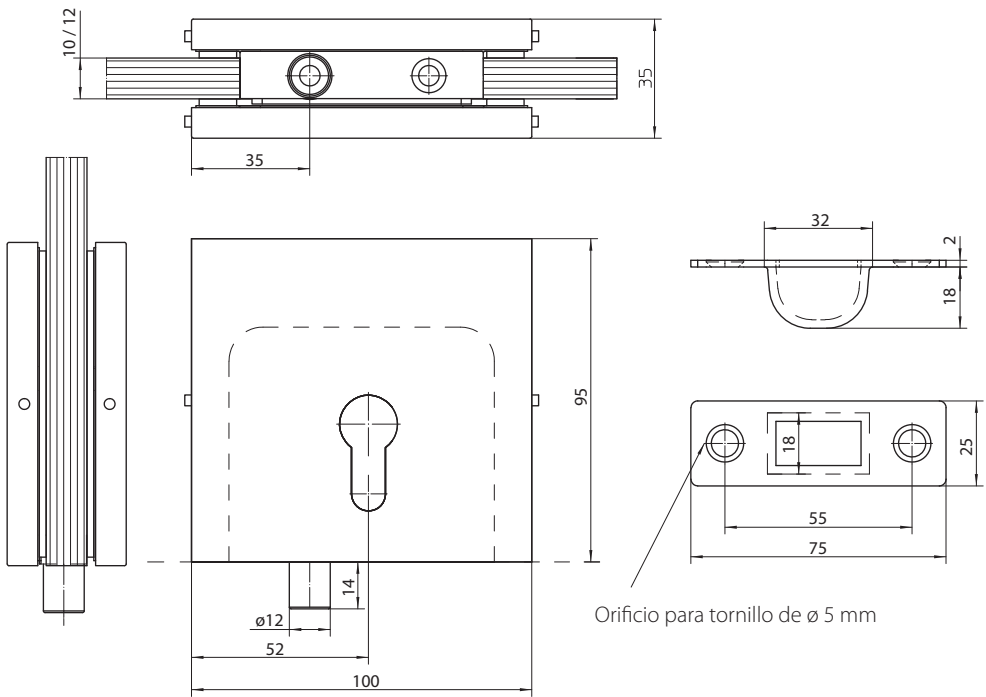
Dibujo nº 91905-1-0118
