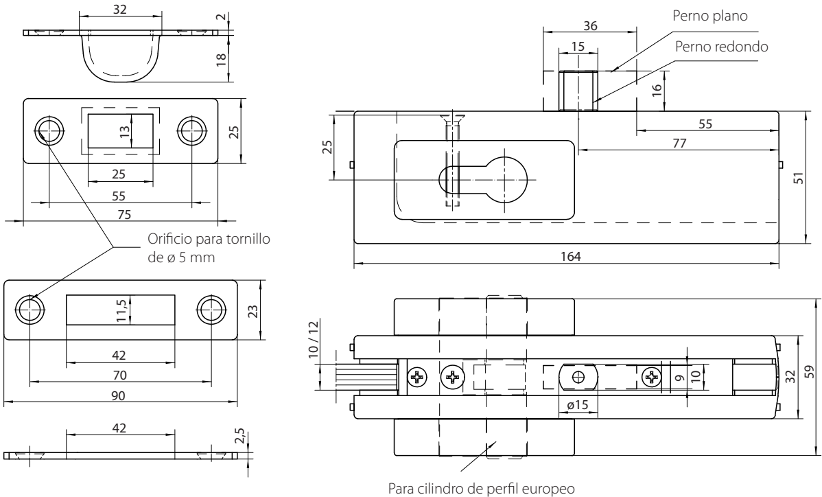
Dibujo nº 91905-1-0117
