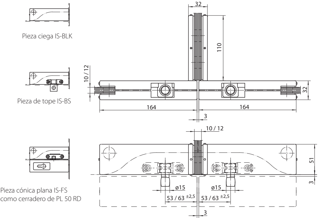
Dibujo nº 91905-1-0108
