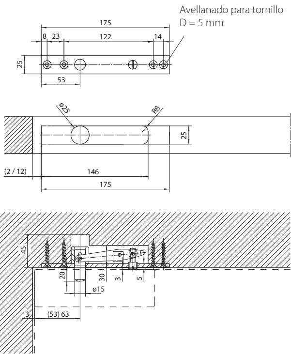
GEZE PT 21 Dibujo nº 91905-1-0102
