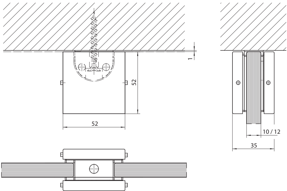
Dibujo nº 91905-1-0116
